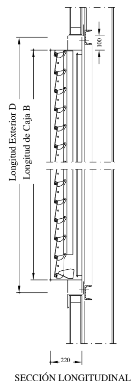
SECCIÓN LONGITUDINAL
